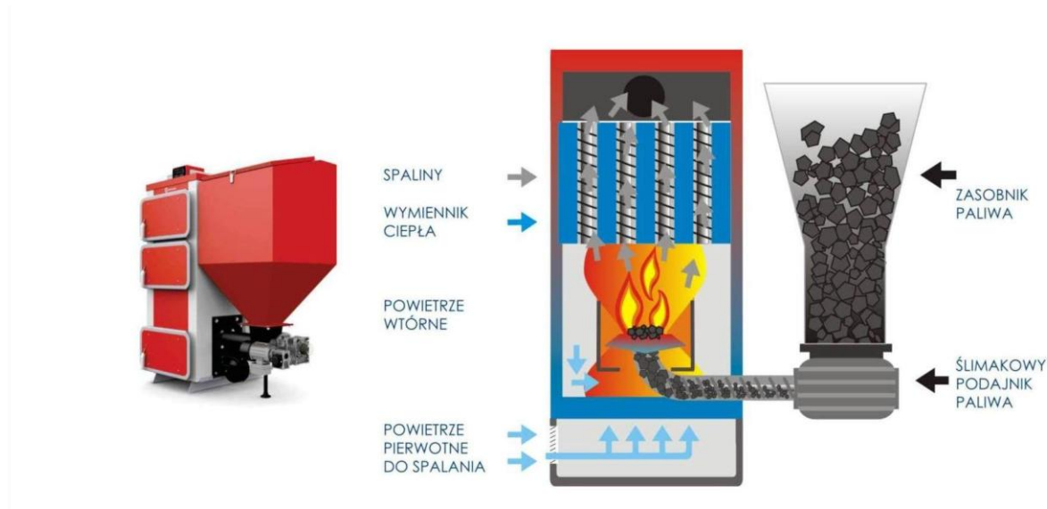
Rysunek 19. Przekrój nowoczesnego kotła retortowego
