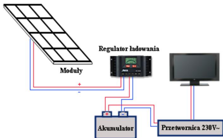
Rysunek 23. Typowy zestaw systemu fotowoltaicznego
