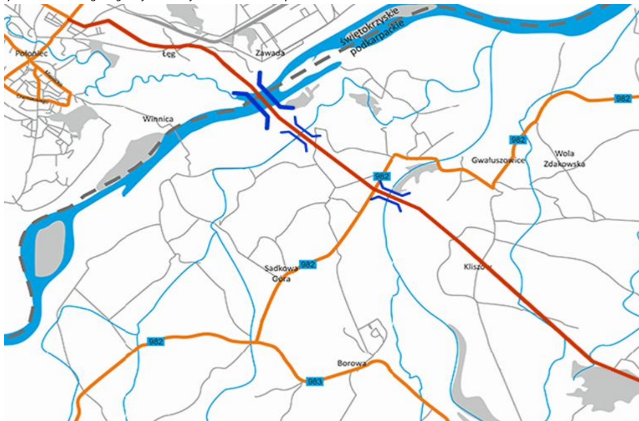
Rysunek 3. Przebieg drogi wojewódzkiej nr 764 wraz z nowym mostem na rzece Wiśle
